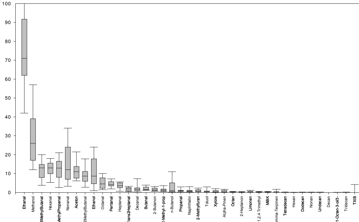
Abb. 4: Verteilung der Konzentrationen an VOC im Hausstaub
