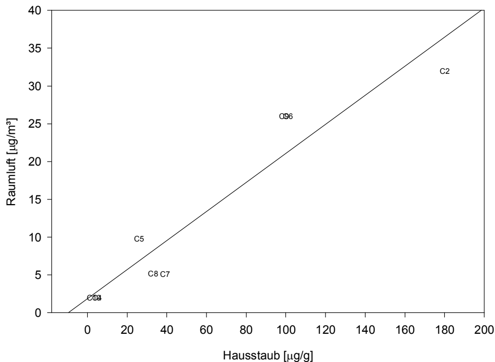
Abb. 6: Zusammenhang zwischen Aldehyd-Belastung der Raumluf und der des Hausstaubes
